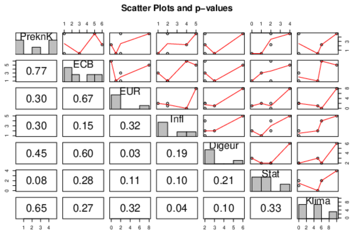
Slika 12: Dijagram rasipanja
